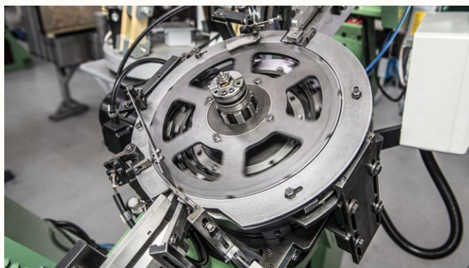
RP8/LD con slitta a pattini in combinazione con caricatore boccole speciale. Caricamento e rullatura boccole fino a 16 mm di diametro.
